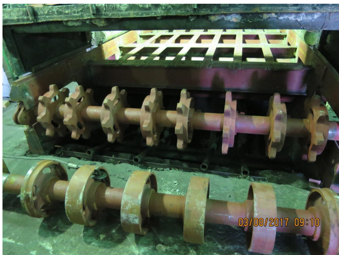
Замена топки котла №4
